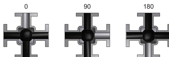
FLOW PLAN 15 4 Way T-Port - 180°
